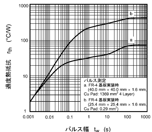
図 7.12 r_{th} - t_w
