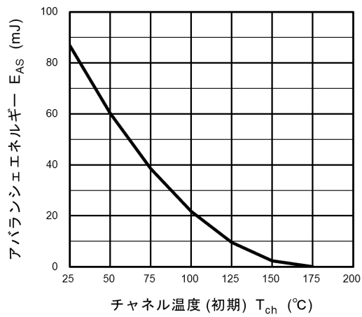
チャネル温度 (初期) T_{ch} ( ^\circ\text{C} ) 図 8.15 E_{AS} - T_{ch} (最大値 (保証値))
