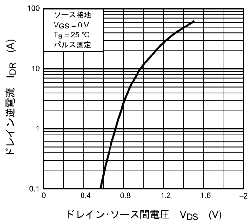
図 8.8 I_{DR} - V_{DS}
