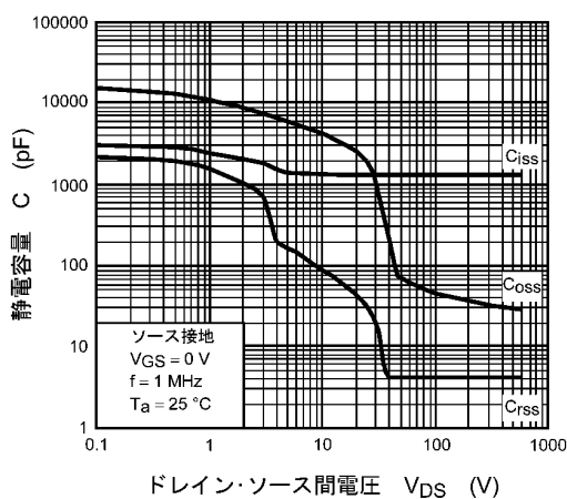
図 8.9 C - V_{DS}
