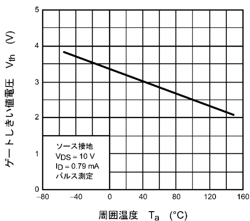
図 8.11 V_{th} - T_a
