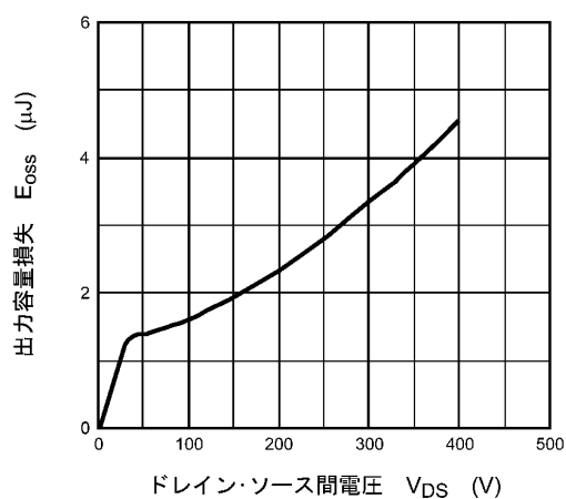
図 8.10 E_{oss} - V_{DS}
