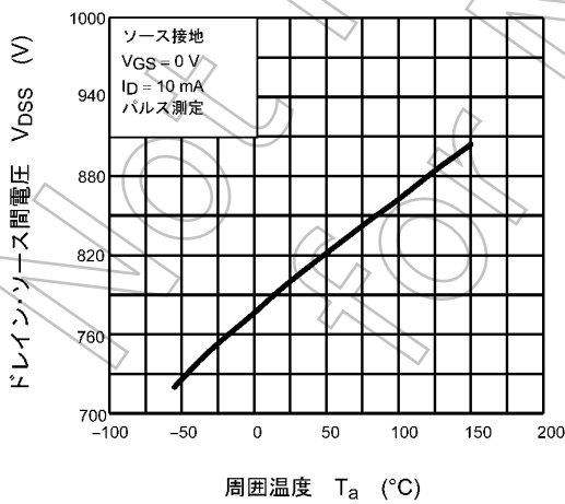
図 8.5 V_{DS} - T_a
