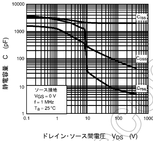
図 8.9 C - V_{DS}
