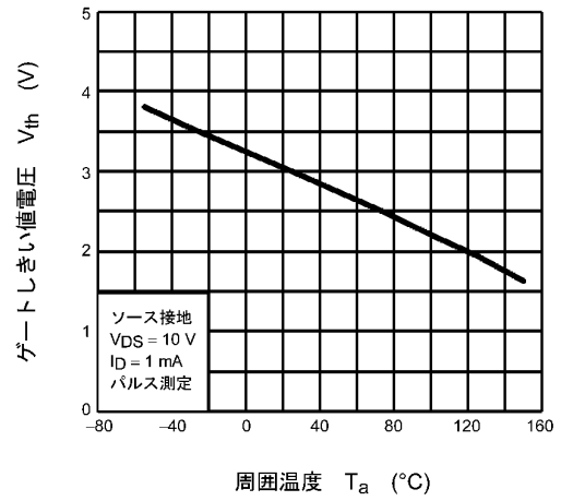
図 8.10 V_{th} - T_a
