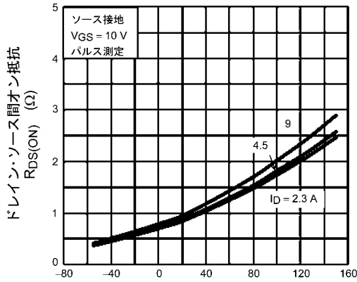
図 8.7 R_{DS(ON)} - T_a
