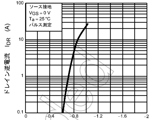
図 8.8 I_{DR} - V_{DS}
