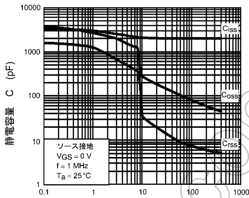
図 8.9 C - V_{DS}
