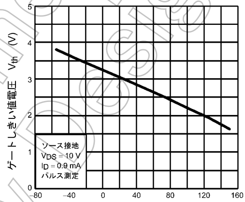
図 8.10 V_{th} - T_a
