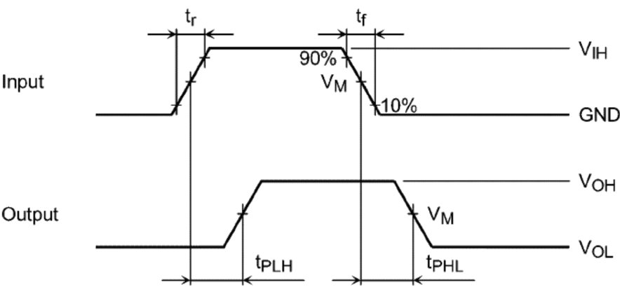
図 9.7.1 AC電氣の特性測定波形
