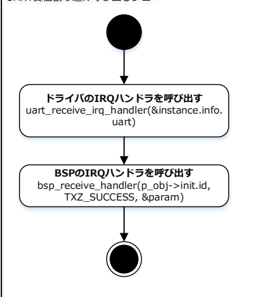
UART受信割り込み呼び出しフロー
