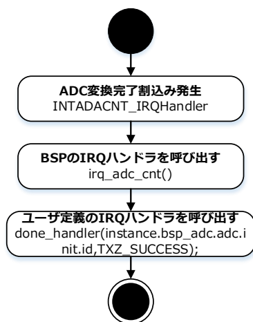
割り込み呼び出しフロー
