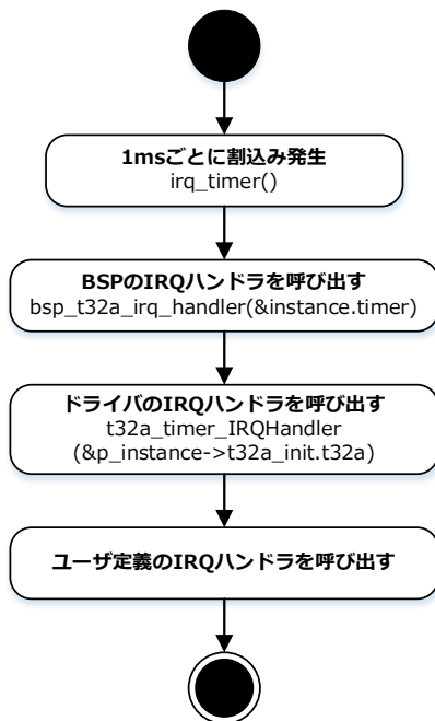
割り込み呼び出しフロー
