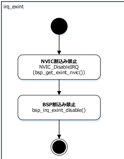
irq_exint
