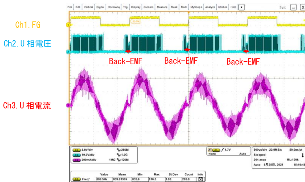
図 1.2 モーター動作の誘起電圧 (Back-EMF) 波形
