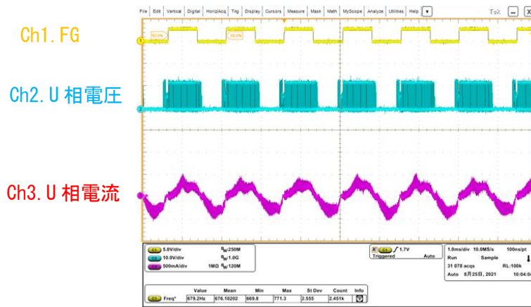
図 1.3 進角 0° モーター動作波形
