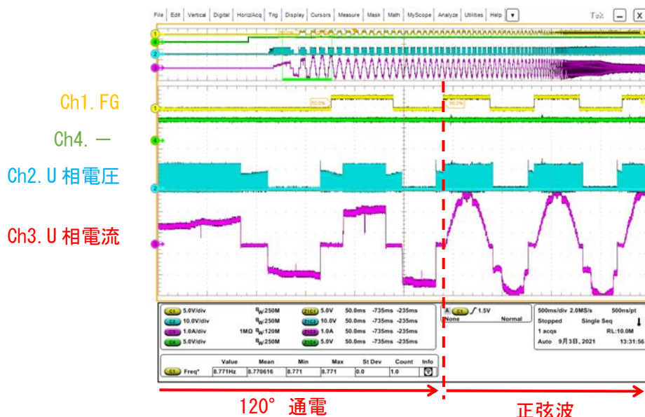
図 1.1 モーター動作の起動時の波形
