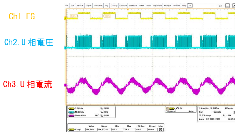
図 1.4 進角 7.5° モーター動作波形
