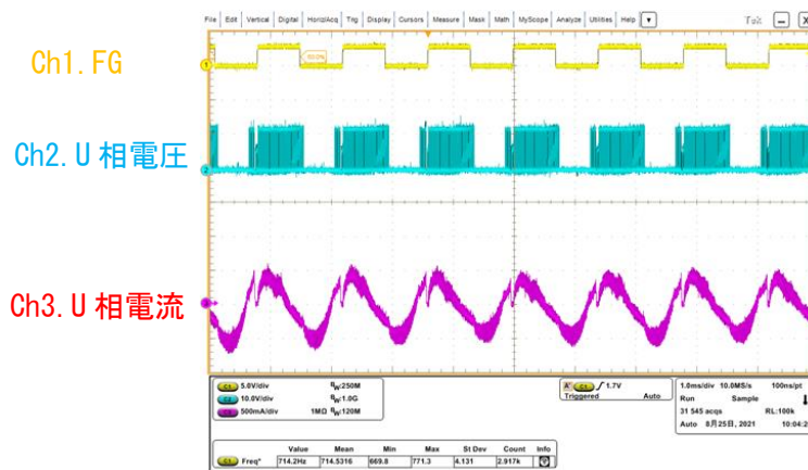
図 1.5 進角 15° モーター動作波形
