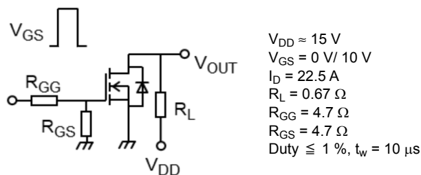
図 6.2.1 スwitching時間の測定回路図
