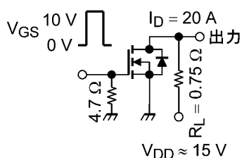
図 6.2.1 スwitching時間の測定回路
