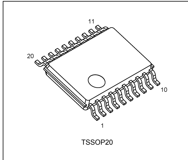
TC74ACT640FT
