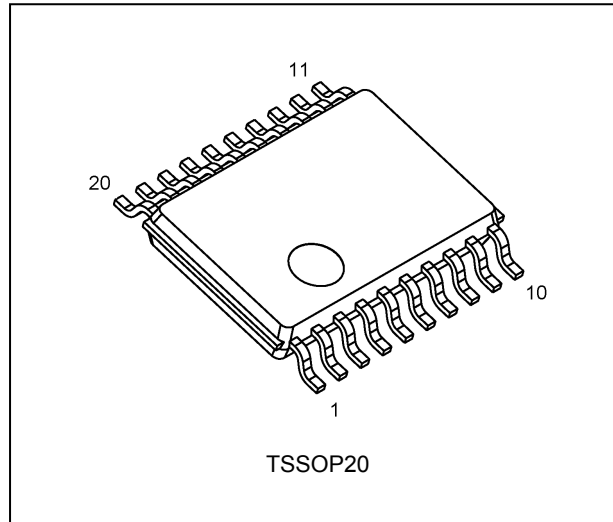
TC74ACT640FT
