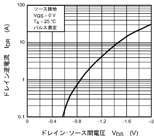
図 8.8 I_{DR} - V_{DS}
