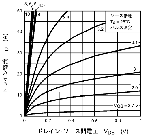
図 8.1 I_D - V_{DS}
