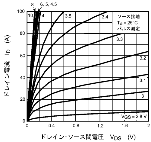
図 8.2 I_D - V_{DS}
