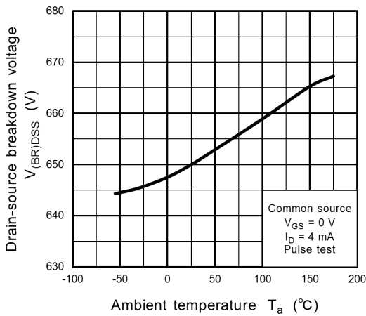
Fig. 8.11 V_{DSS} - T_a
