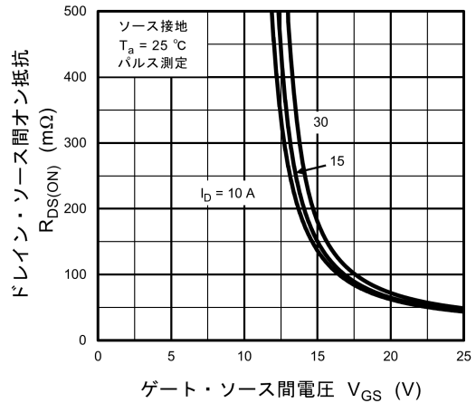
図 8.8 R_{DS(ON)} - V_{GS}
