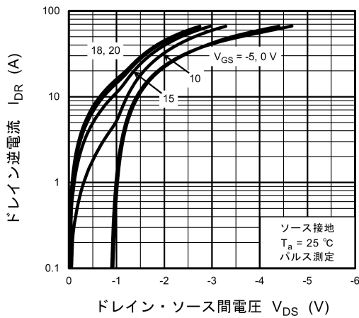
図 8.9 I_{DR} - V_{DS}
