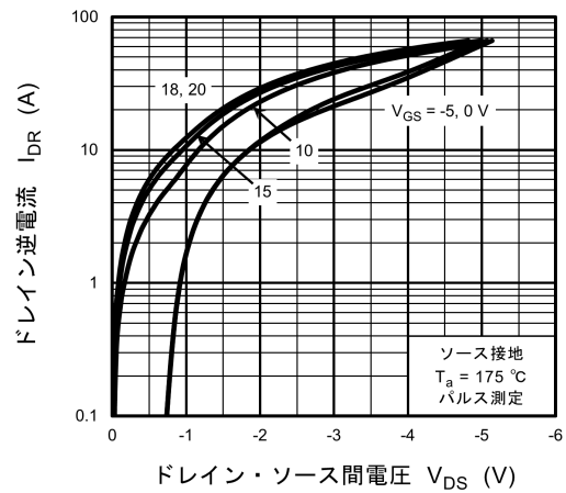
図 8.10 I_{DR} - V_{DS}
