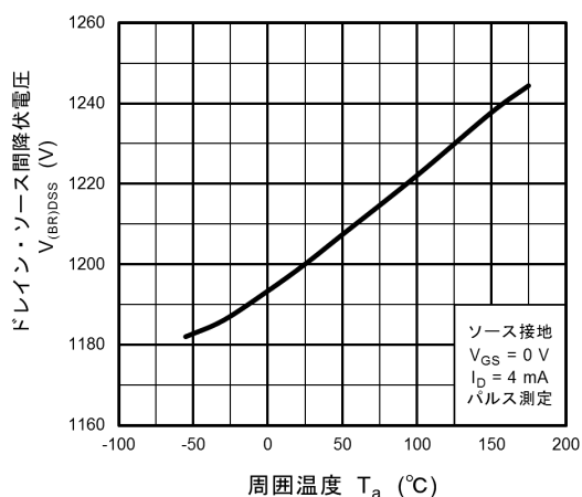
図 8.11 V_{DSS} - T_a
