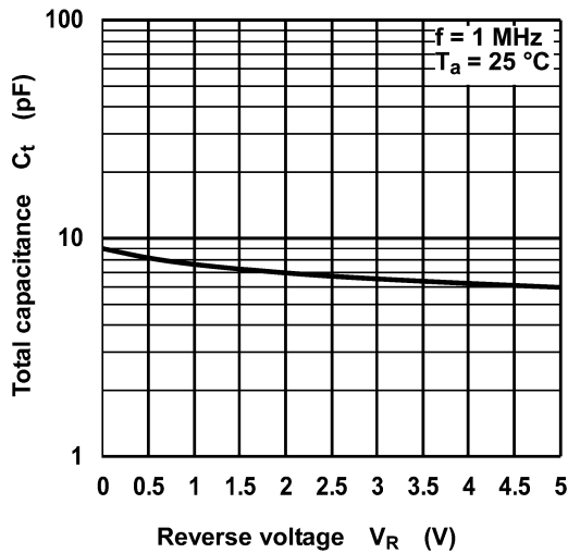
図 8.3 C_t - V_R
