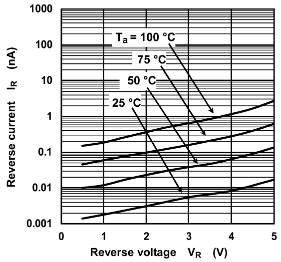
図 8.2 I_R - V_R
