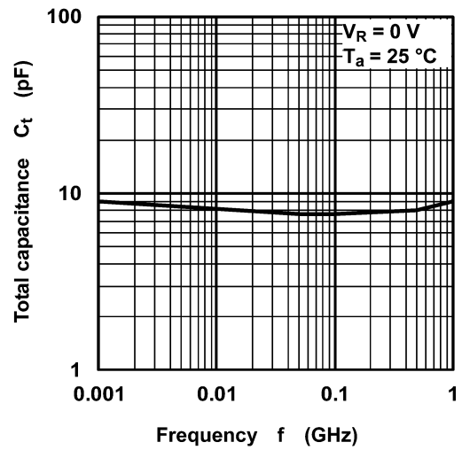
図 8.4 C_t - f
