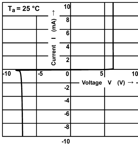
図 8.1 I - V
