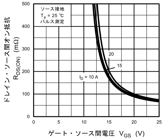
図 8.8 R_{DS(ON)} - V_{GS}
