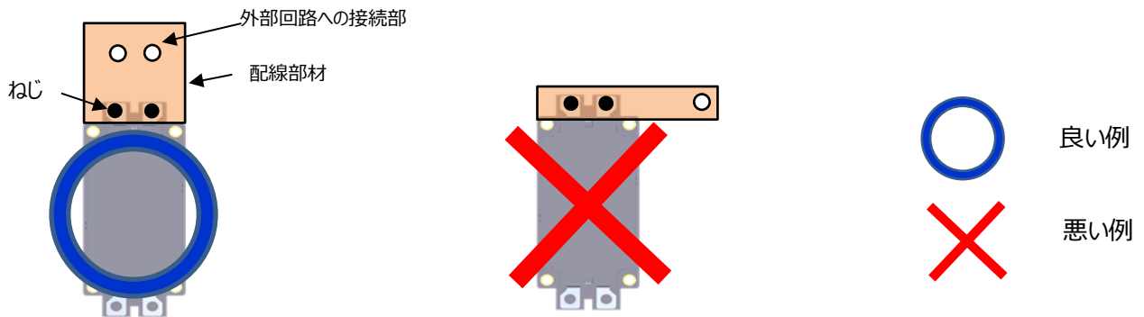
図 2.5.2 主端子と主回路配線部材の設計例(AC端子の接続例)
