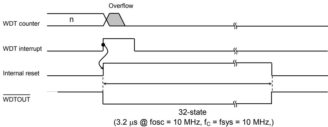
Fig. 16-3 Reset Mode
