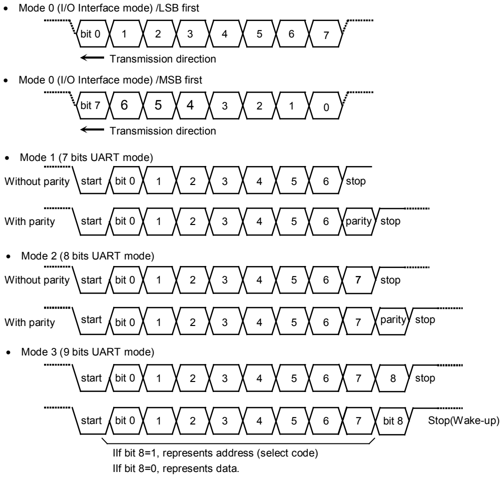
Fig. 11-1 Data Format
