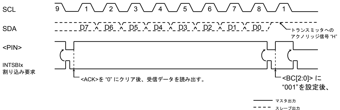
図 12-17 マスタレシーバモード時、データの送信を終了させるときの処理
