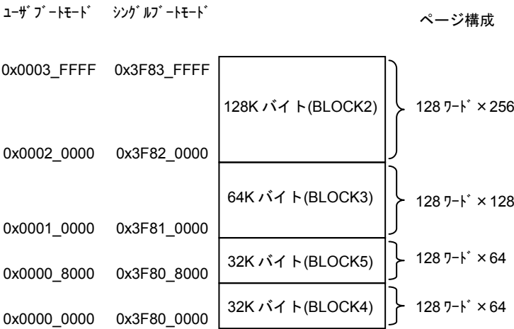
図 18-9 フラッシュメモリのブロック構成
