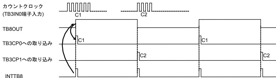
図 10-7 周波数測定
