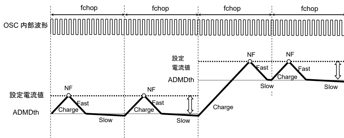
図 6.18 設定電流値が増加方向の場合
