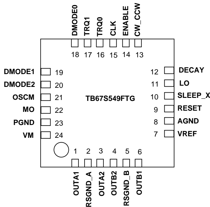
图 4.1 端子配置图
