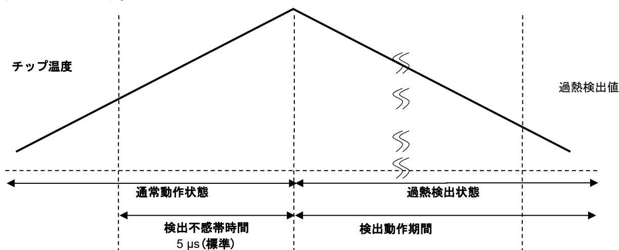
図 6.25 過熱検出
