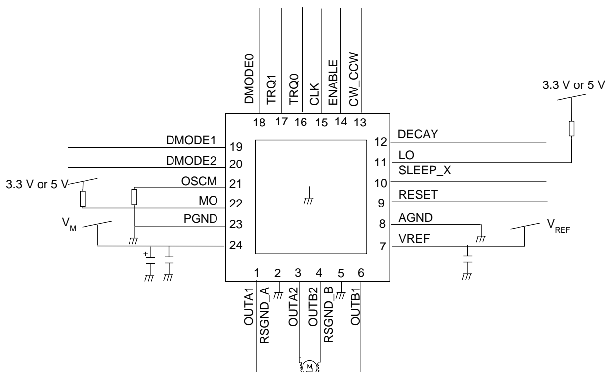
図 10 応用回路例
