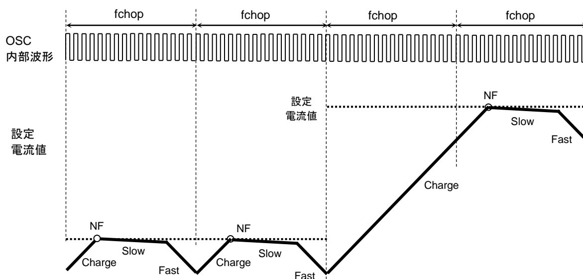
図 6.13 Charge 期間が f_{chop} 1 周期以上の場合
