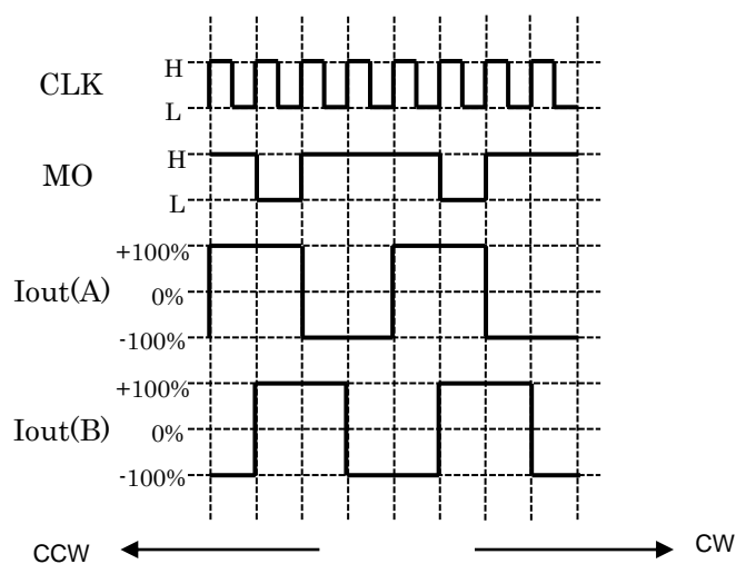
図 6.1 2 相励磁設定
