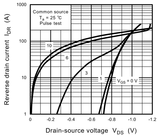
Fig. 8.6 I_{DR} - V_{DS}
