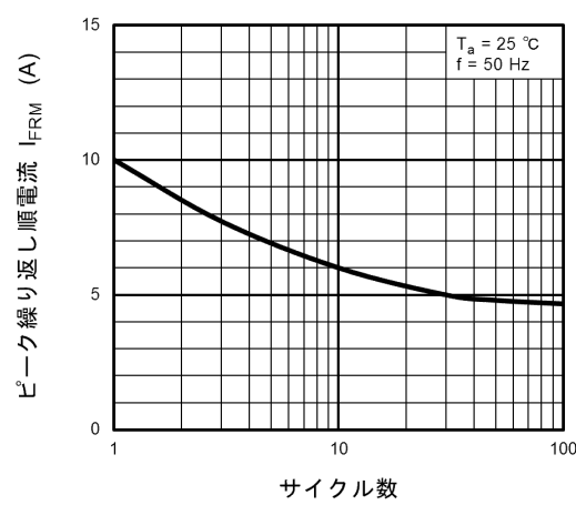
図 10.6 I_{FRM} - \text{サイクル数} (最大値)
