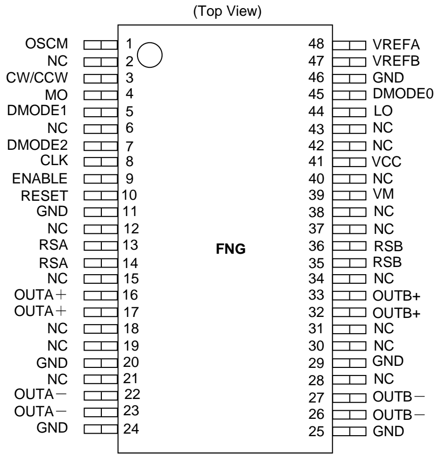
図 4.2 ピン配置図(FNG)
