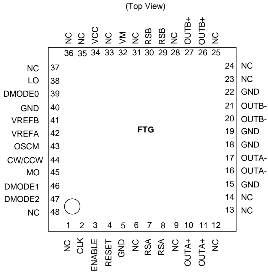
図 4.1 ピン配置図(FTG)
