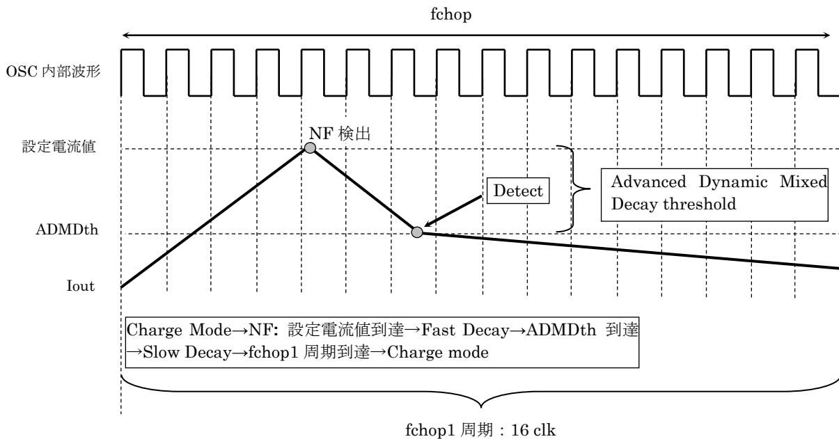
図 6.9 ADMD 定電流制御
