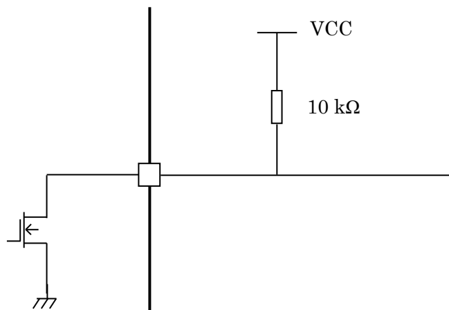
図 6.8 LO 端子
