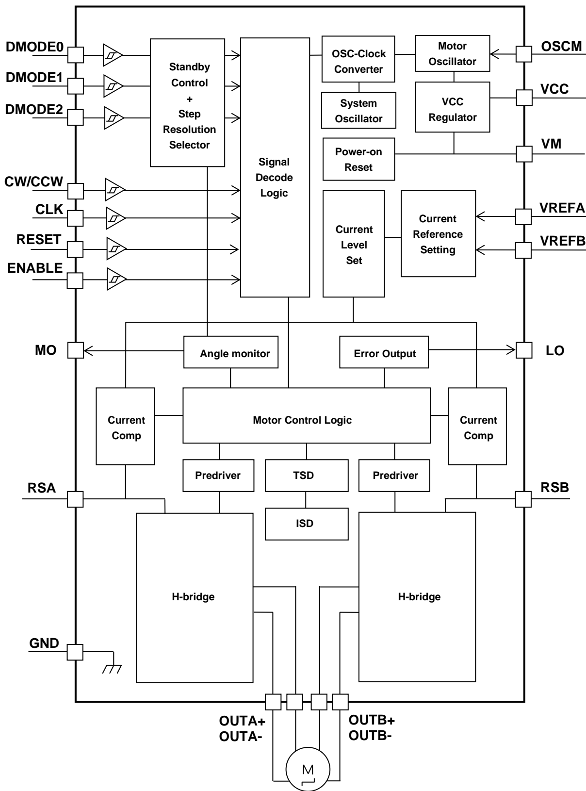
図 3.1 TB67S109A ブロック図
