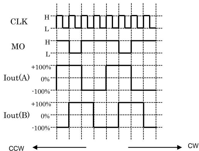
図 6.1 2 相励磁設定
