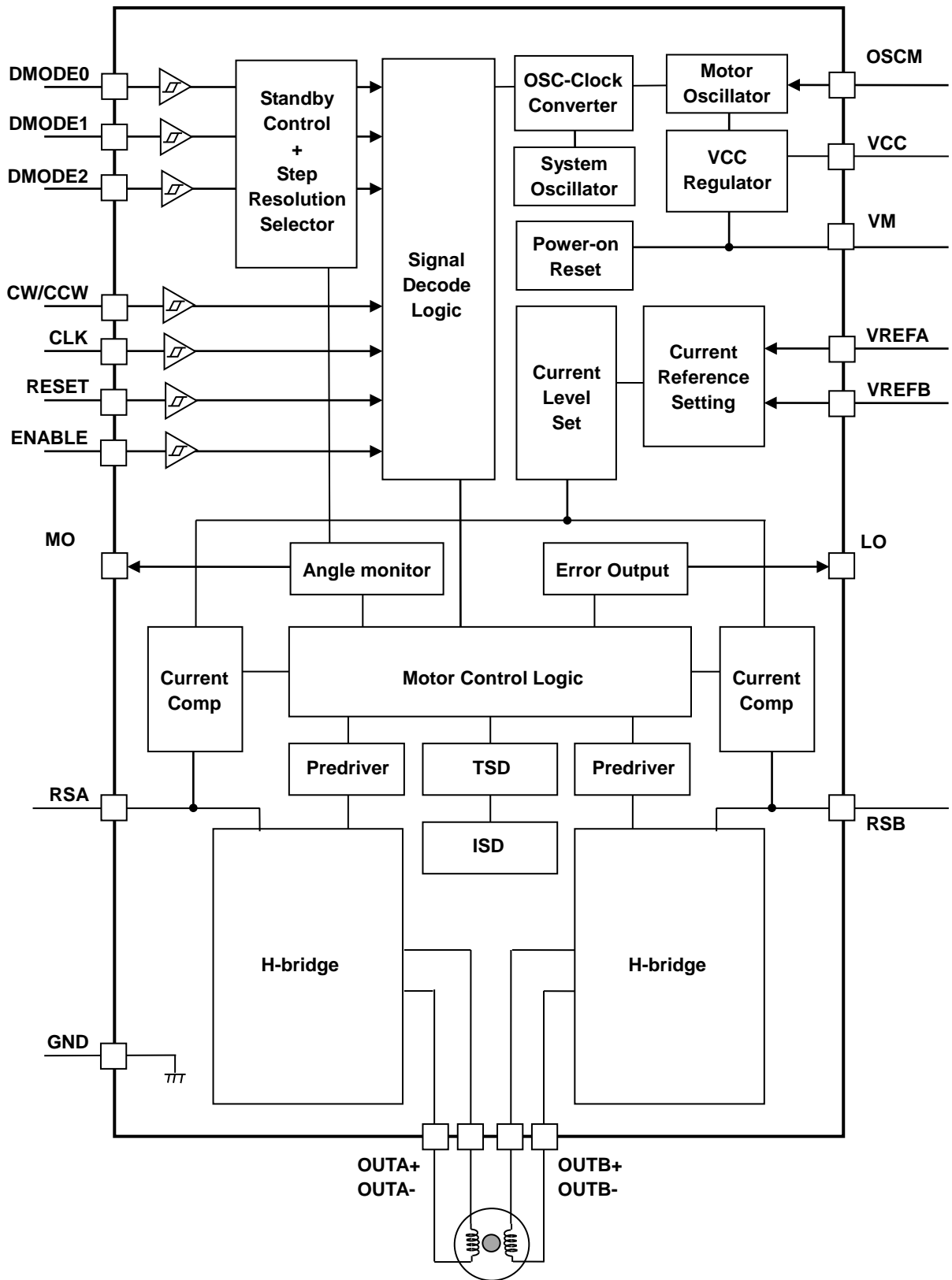
TB67S109A ブロック図
