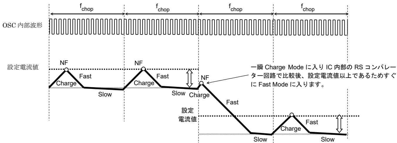
図 6.13 設定電流値が減少方向の場合
