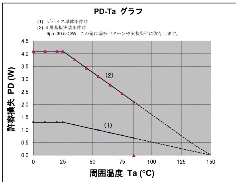
図 9.2 許容損失と周囲温度の関係
