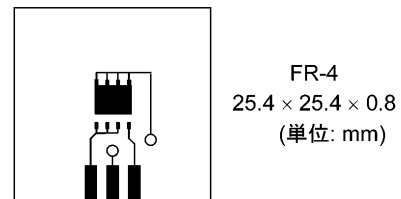
図 5.2 ガラスエポキシ基板 実装例b
