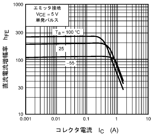
図 7.3 h_{FE} - I_C
