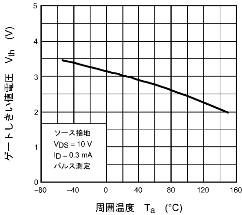
図 8.9 V_{th} - T_a
