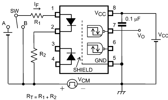
図 12.1.6 コモンモード過渡耐性測定回路, 波形
