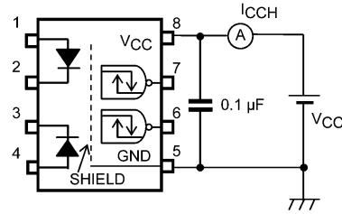
図 12.1.4 ICCH測定回路
