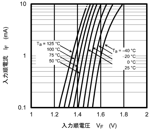
図 12.2.1 I_F - V_F
