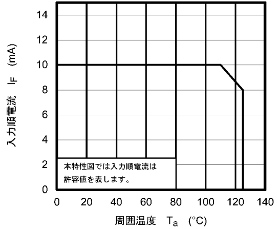
図 12.2.2 I_F - T_a
