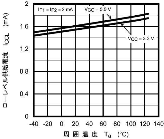
図 12.2.7 I_{CCL} - T_a
