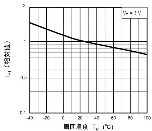
図 12.6 相対 I FT - T a
