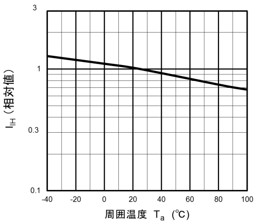
図 12.11 相対 I_{IH} - T_a
