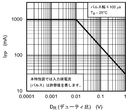
図 12.4 I FP - D R
