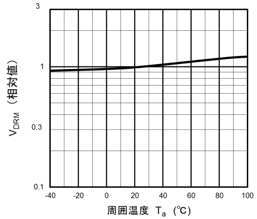
図 12.8 相対 V_{DRM} - T_a
