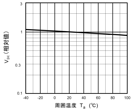
図 12.10 相対 V_{IH} - T_a
