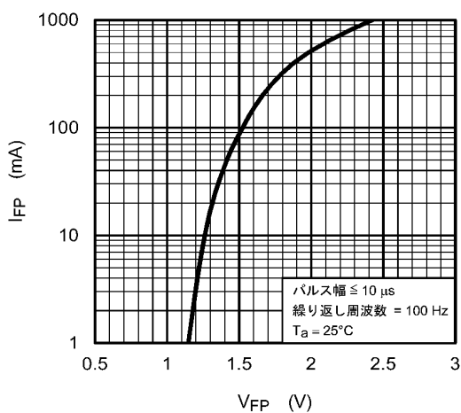
図 12.5 I FP - V FP
