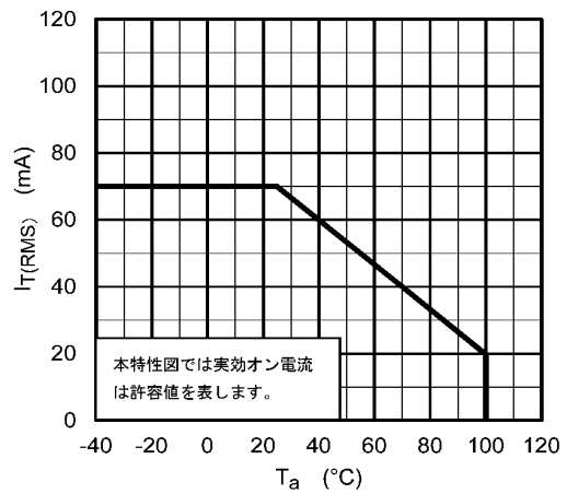
図 12.2 I T(RMS) - T a
