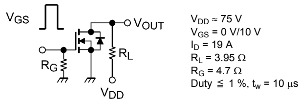
図 6.2.1 スwitchング時間の測定回路
