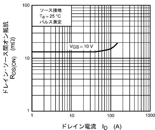
図 8.5 R_{DS(ON)} - I_D
