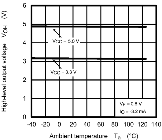
Fig. 12.2.6 V_{OH} - T_a
