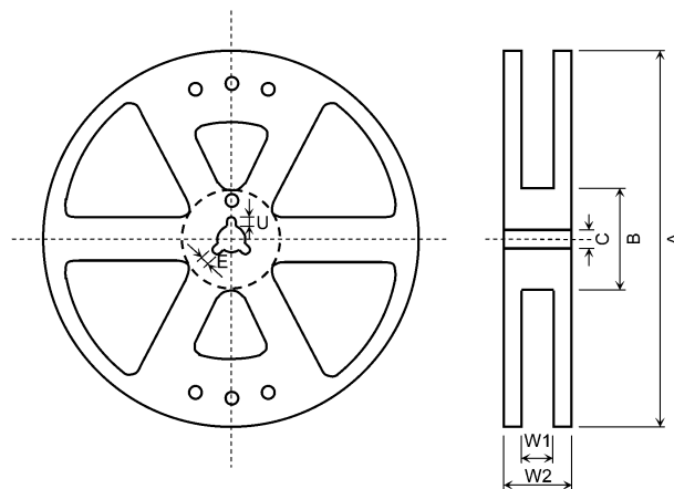
図 17.3.6.1 リール形状
