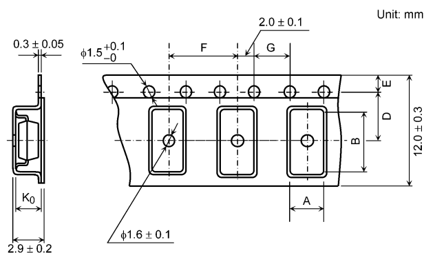
図 17.3.5.1 テーピング形状
