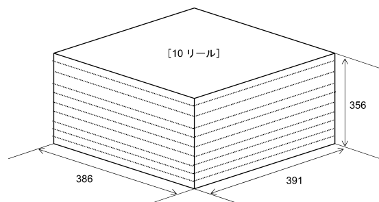
図 17.4.2 10リール入り梱包箱 (unit: mm)
