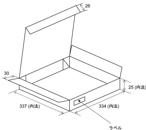
図 17.4.1 1リール入り梱包箱 (unit: mm)
