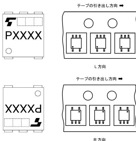
図 17.3.1.1 凹み角穴内の製品の向き
