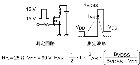
測定回路 測定波形 図 8.16 測定回路/測定波形
