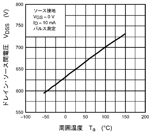
図 8.5 V_{DS} - T_a
