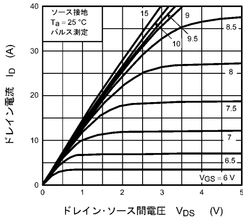
図 8.1 I_D - V_{DS}
