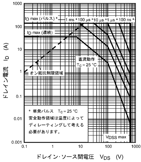
図 8.17 安全動作領域 (最大値 (保証値))
