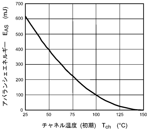
チャンネル温度 (初期) T_{ch} (°C) 図 8.14 E_{AS} - T_{ch} (最大値 (保証値))
