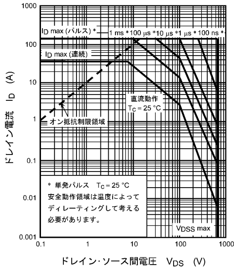
図 8.17 安全動作領域 (最大値 (保証値))
