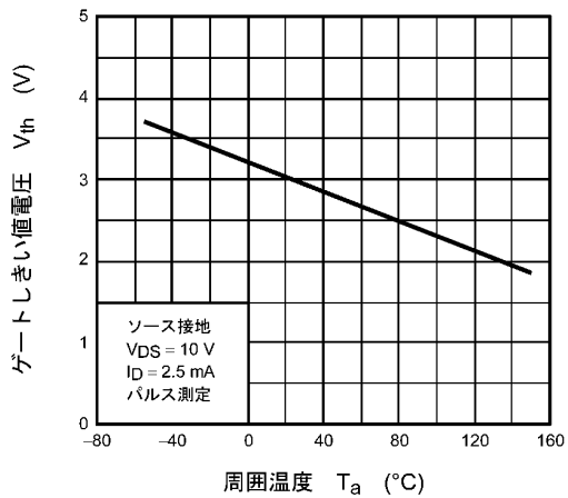
図 8.11 V_{th} - T_a
