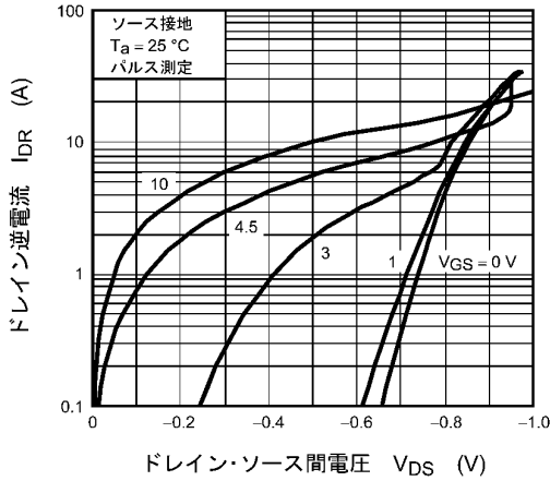
図 8.7 I_{DR} - V_{DS}
