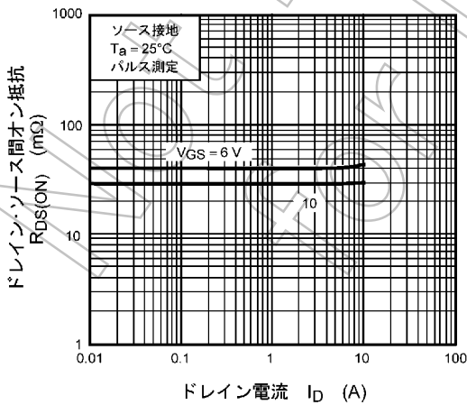
図 8.1.5 R_{DS(ON)} - I_D
