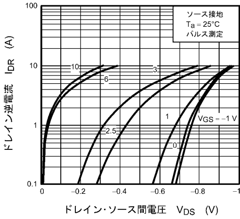
図 8.1.7 I_{DR} - V_{DS}
