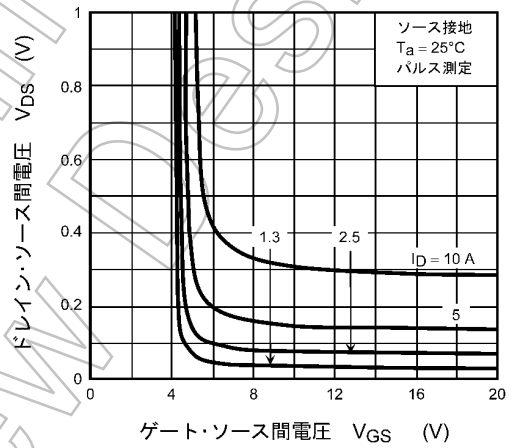
図 8.1.4 V_{DS} - V_{GS}
