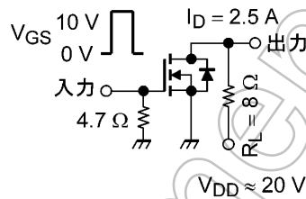
図 6.2.1.1 スイッチング時間の測定回路例
