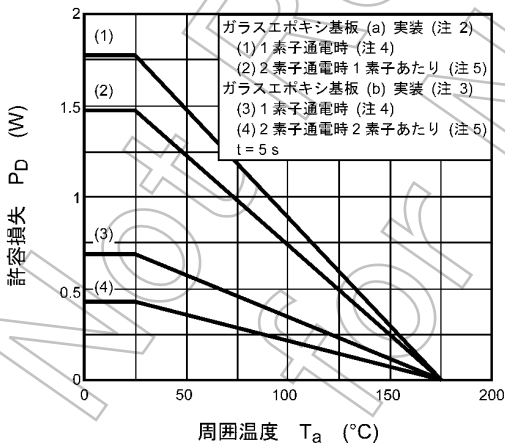
図 8.1.11 P_D - T_a (最大値 (保証値)) (注10)
