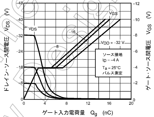
図 8.2.10 ダイナミック入出力特性
