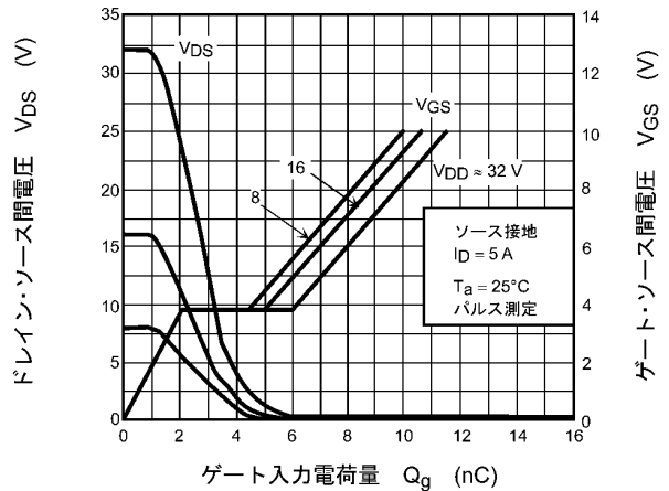
図 8.1.10 ダイナミック入出力特性
