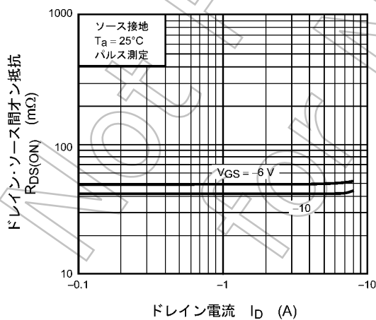
図 8.2.5 R_{DS(ON)} - I_D
