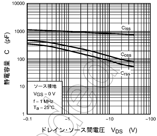
図 8.2.8 静電容量 - V_{DS}
