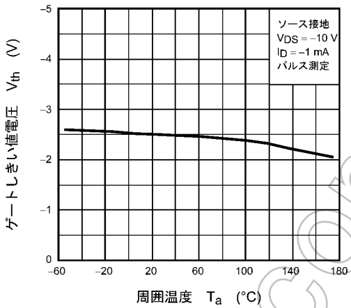
図 8.2.9 V_{th} - T_a (注10)
