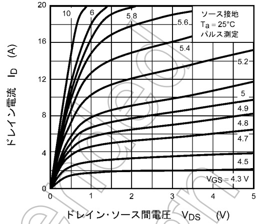
図 8.1.2 I_D - V_{DS}
