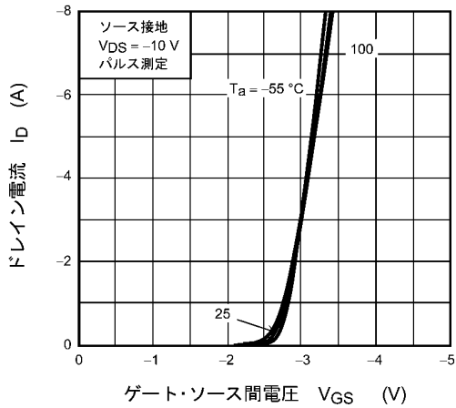
図 8.2.3 I_D - V_{GS}
