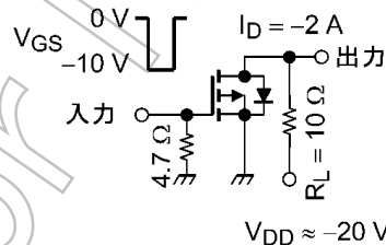
図 6.2.2.1 スイッチング時間の測定回路例
