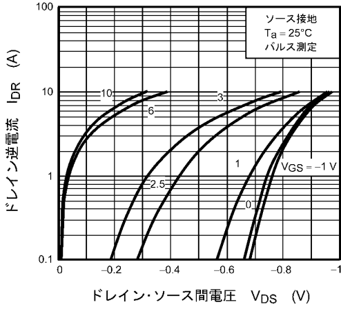
図 8.1.7 I_{DR} - V_{DS}
