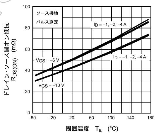
図 8.2.6 R_{DS(ON)} - T_a (注10)
