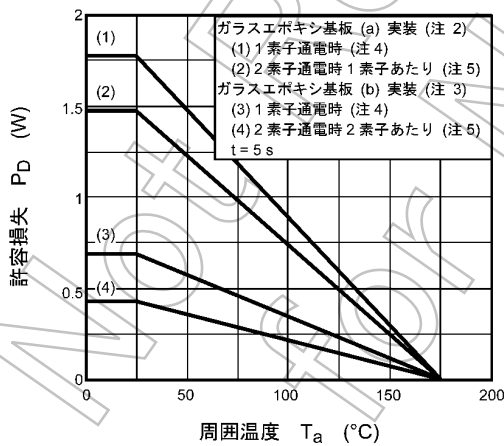
図 8.2.11 P_D - T_a (最大値 (保証値)) (注10)
