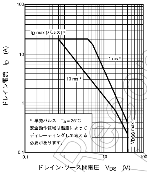
図 8.1.13 安全動作領域 (最大値 (保証値))
