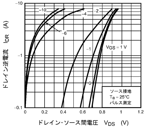
図 8.2.7 I_{DR} - V_{DS}
