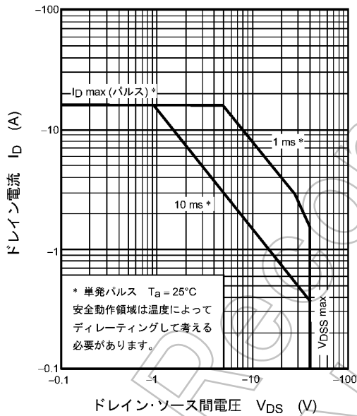
図 8.2.13 安全動作領域 (最大値 (保証値))
