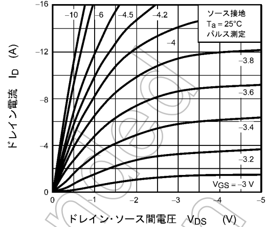
図 8.2.2 I_D - V_{DS}
