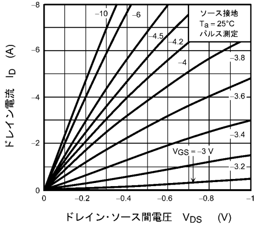
図 8.2.1 I_D - V_{DS}
