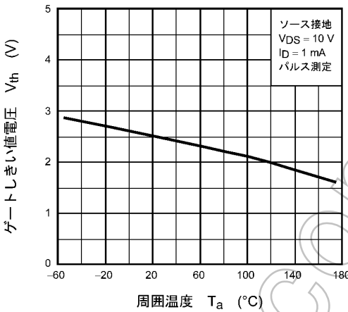
図 8.1.9 V_{th} - T_a (注10)
