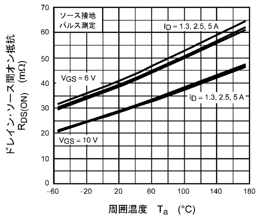
図 8.1.6 R_{DS(ON)} - T_a (注10)
