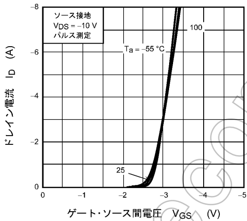
図 8.2.3 I_D - V_{GS}
