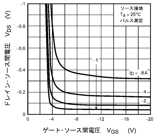
図 8.2.4 V_{DS} - V_{GS}
