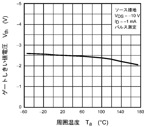
図 8.2.9 V_{th} - T_a (注10)
