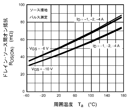
図 8.2.6 R_{DS(ON)} - T_a (注10)
