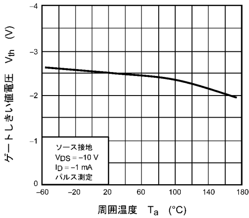
図 8.9 V_{th} - T_a (注8)
