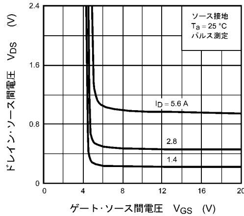
図 8.4 V_{DS} - V_{GS}
