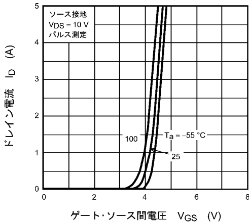
図 8.3 I_D - V_{GS}
