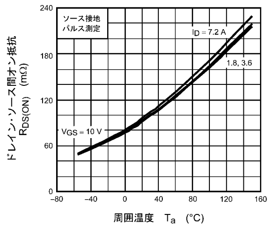
図 8.6 R_{DS(ON)} - T_a
