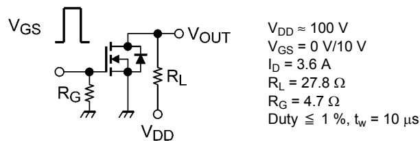
図 6.2.1 スwitching時間の測定回路例
