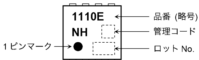
図 7.1 現品表示
