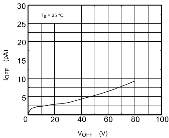
Fig. 12.1.9 I_{OFF} - V_{OFF}
