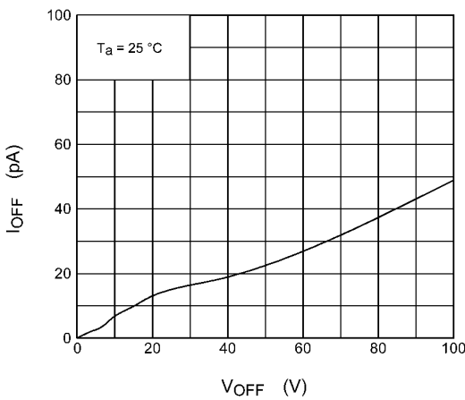
Fig. 12.1.9 I_{OFF} - V_{OFF}
