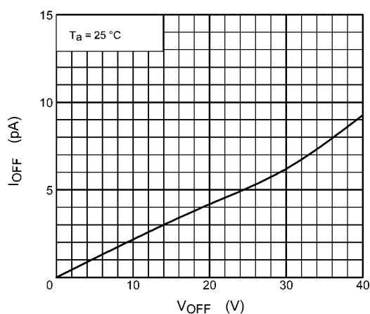
図 12.1.9 I_{OFF} - V_{OFF}
