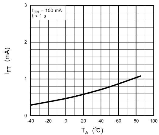
図 12.1.6 I_{FT} - T_a
