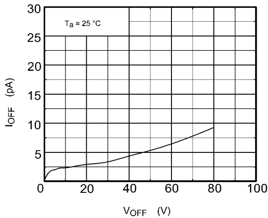
図 12.1.9 I_{OFF} - V_{OFF}
