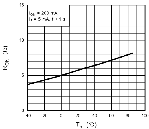
図 12.1.5 R_{ON} - T_a
